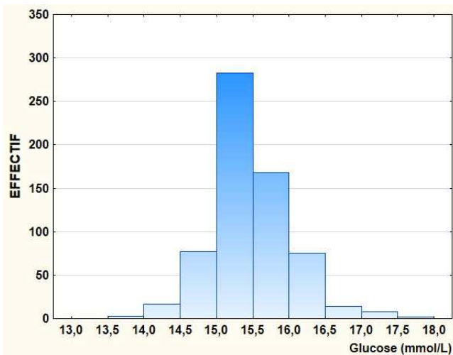
Glucose : échantillon 16S
