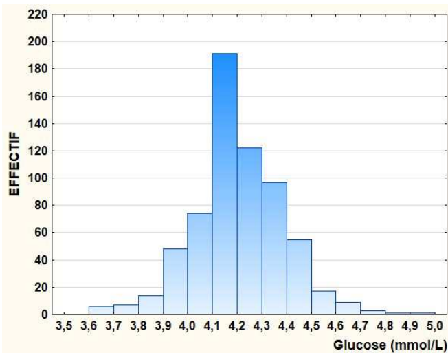
Glucose : échantillon 16R
