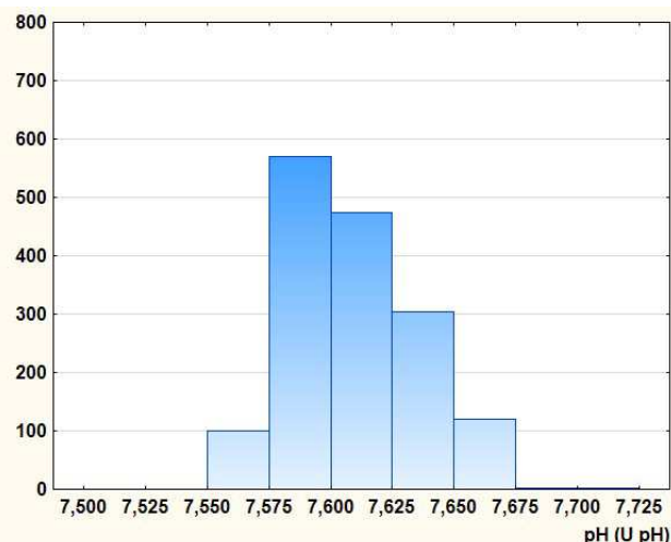
pH : échantillon 16S
