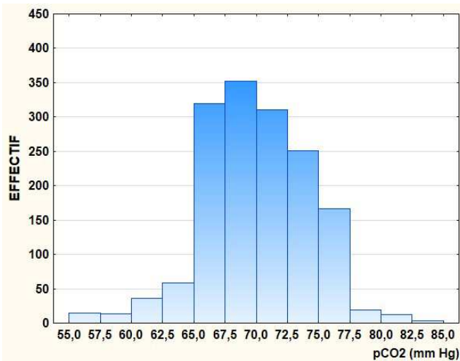
pCO2 : échantillon 16R
